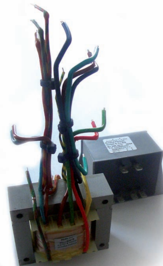
NF - Übertrager mit Verguss
